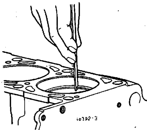
Рис.76. Замер теплового зазора в стыке поршневых колец
