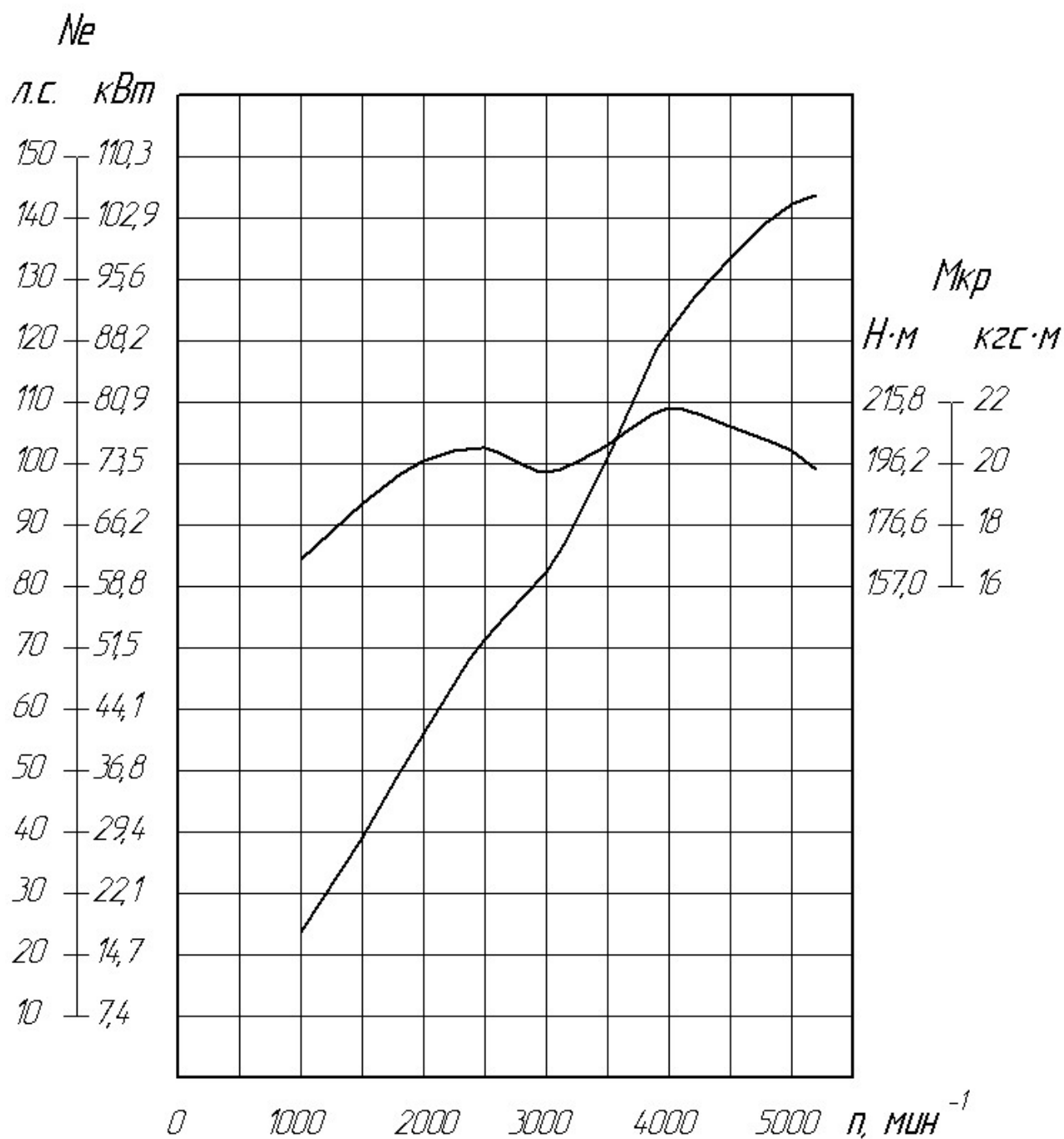
Рис.5. Внешняя скоростная характеристика двигателя
