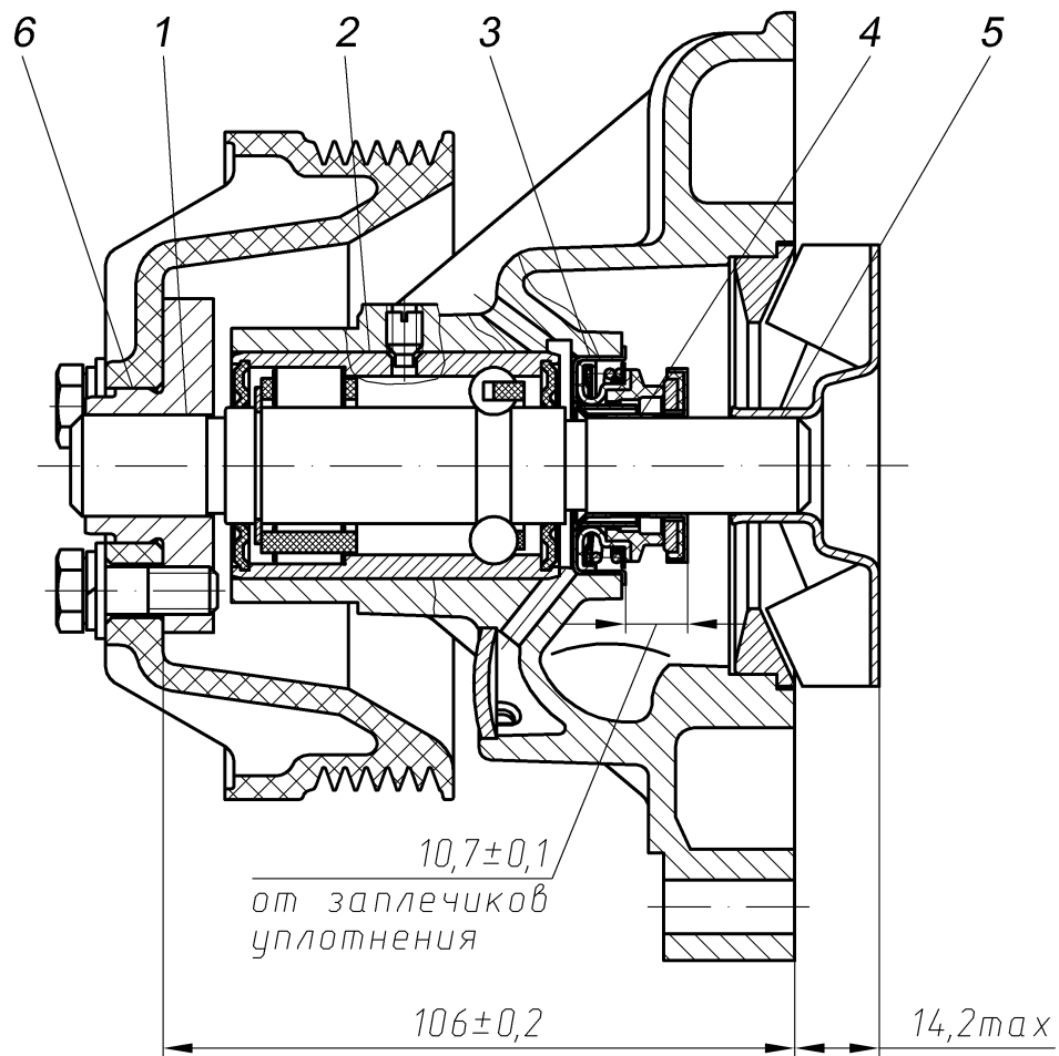
Рис.95. Водяной насос
