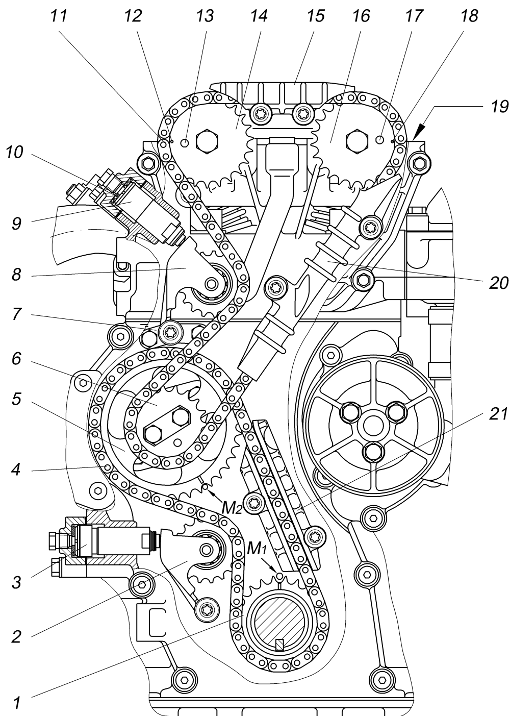
Рис.18. Привод распределительных валов втулочными двухрядными и однорядными цепями:
