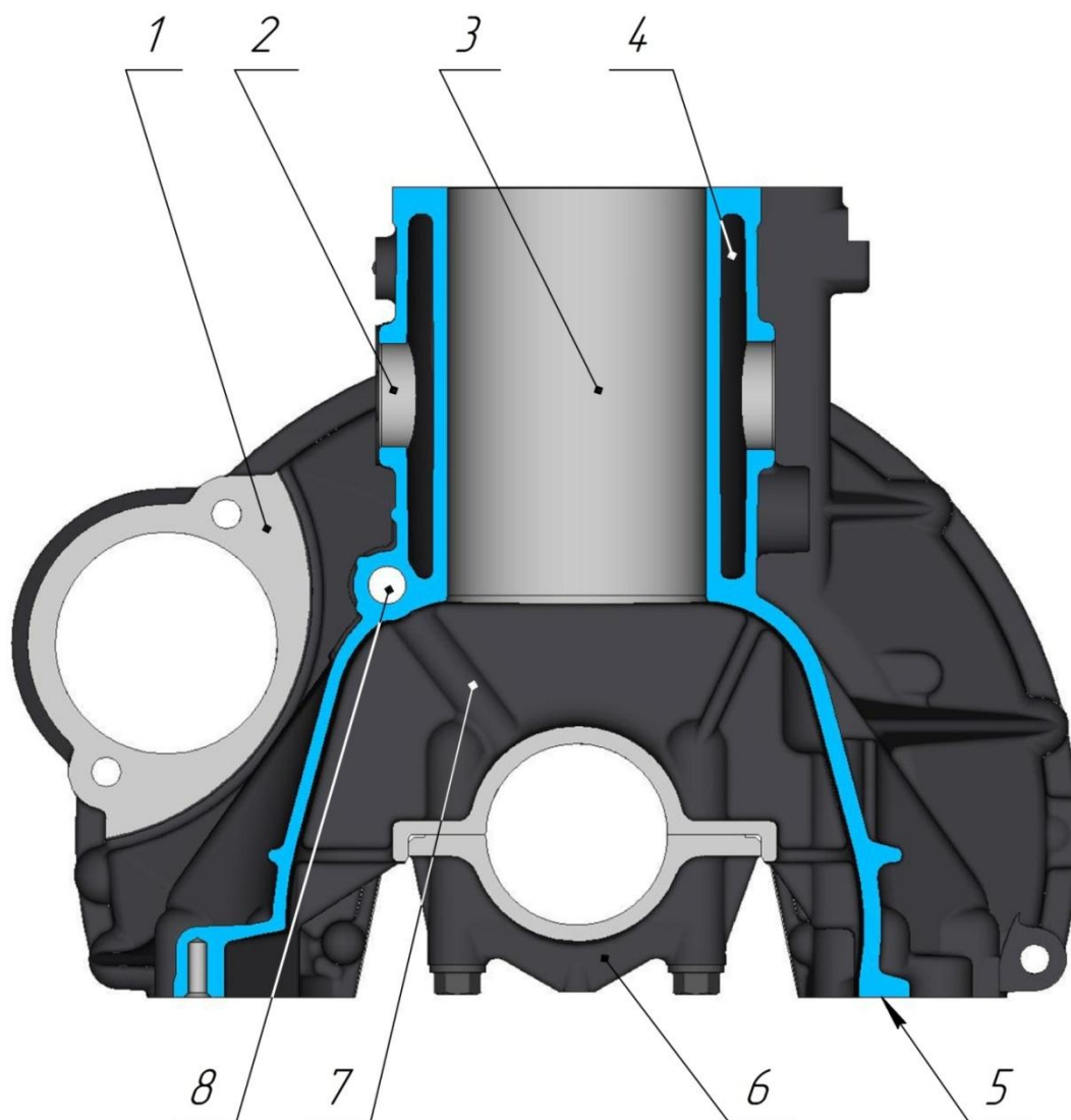
Рис.8. Блок цилиндров. Поперечный разрез по оси цилиндра:
