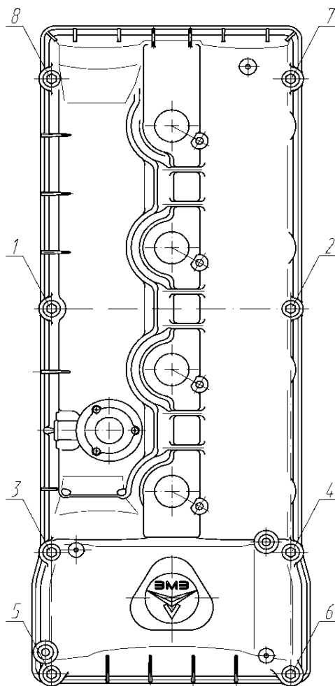
Рис.83. Последовательность затяжки болтов крышки клапанов
