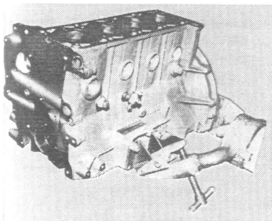
Рис.69. Установка блока цилиндров на стенд
