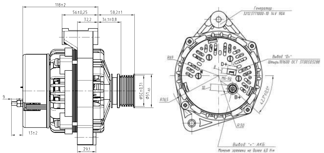
Рис.40. Габаритные размеры генератора 3212.3771000-10 ОАО «БАТЭ» (90А)
