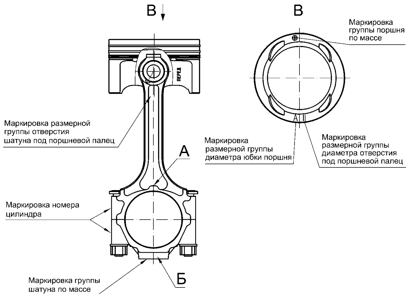
Рис.75. Маркировка шатуна и поршня
