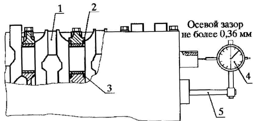
Рис.71. Проверка осевого зазора коленчатого вала:
