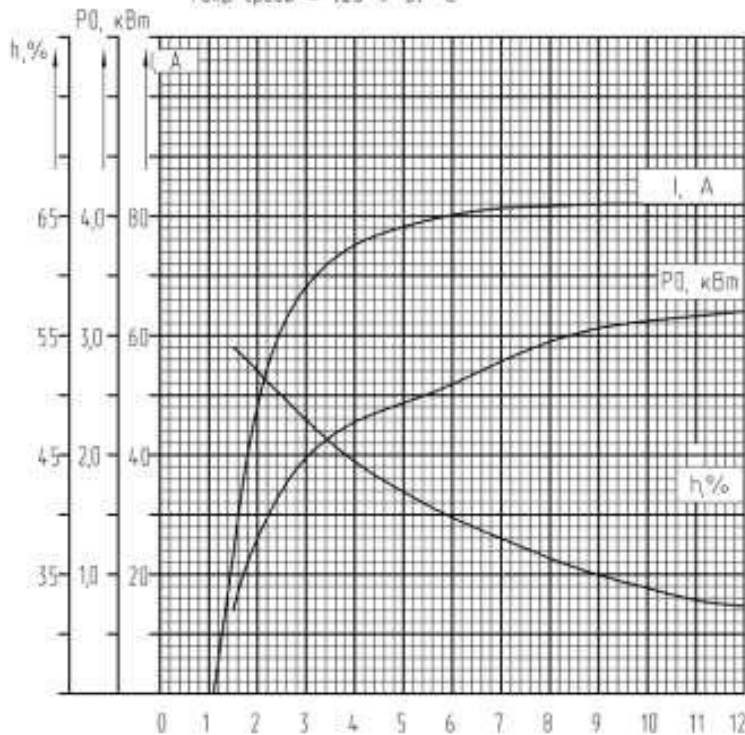
Рис.39. Габаритные размеры и токоскоростная характеристика генераторов 4052.3701000-01 ОАО «Промо-Искра» и 5122.3771000 ООО СП «Промо-Электро» (80А)
