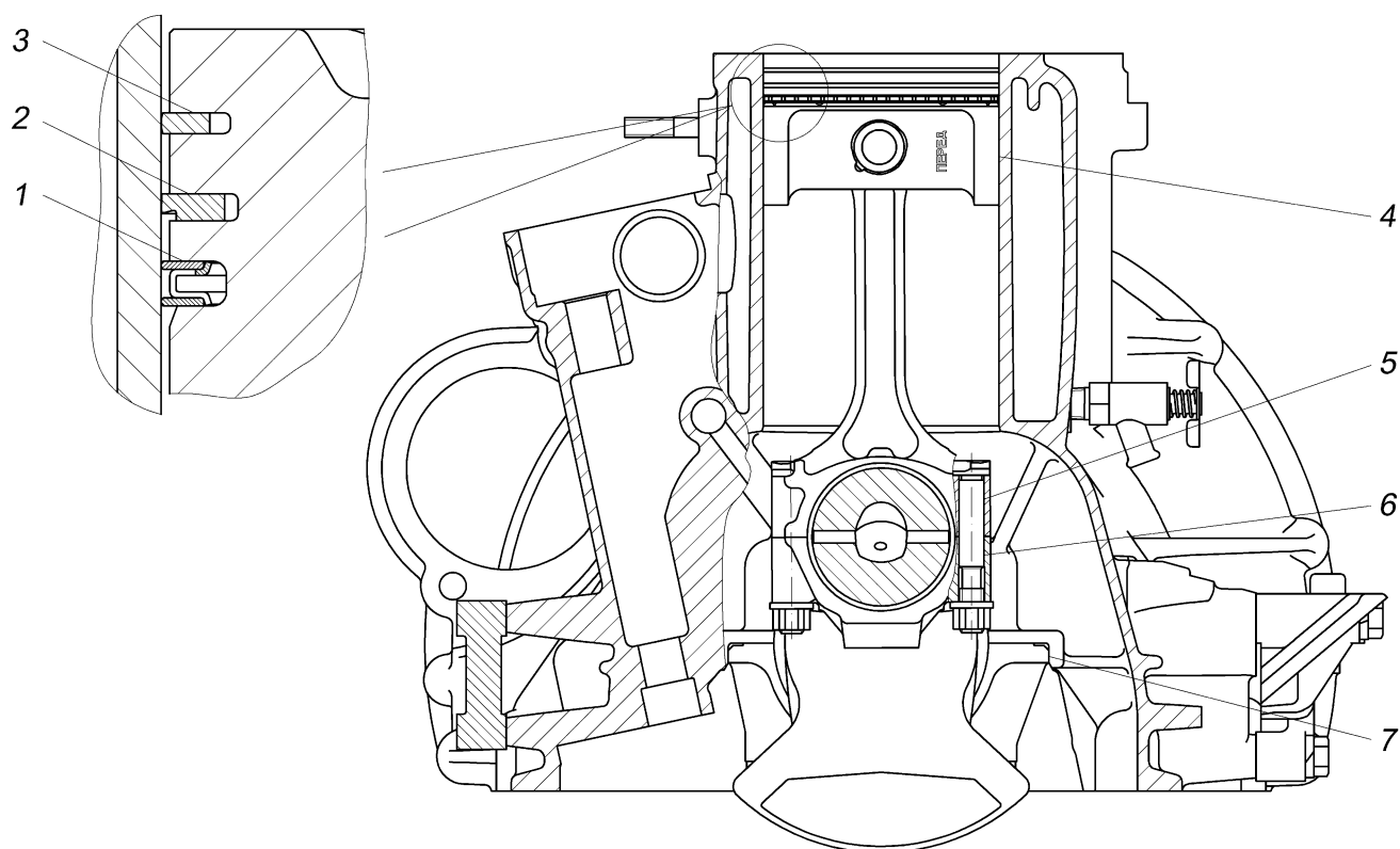
Рис.90. Блок цилиндров и поршень
