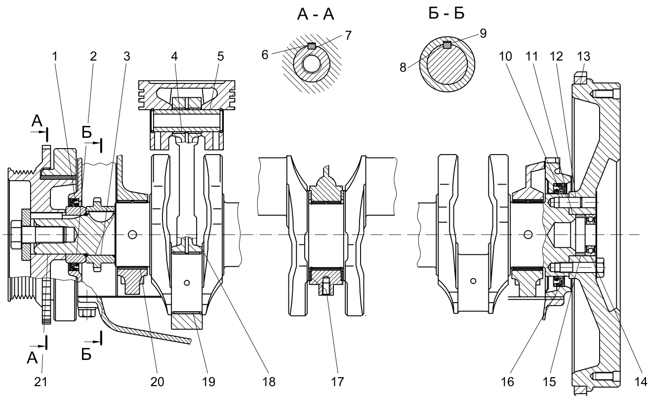
Рис.91. Кривошипно-шатунный механизм
