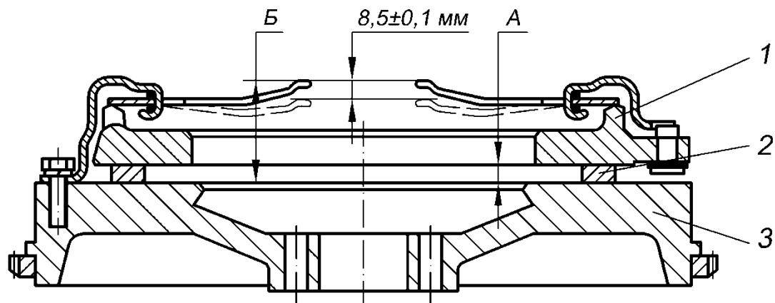
Рис.88. Регулировка концов лепестков и проверка нажимного диска сцепления:
