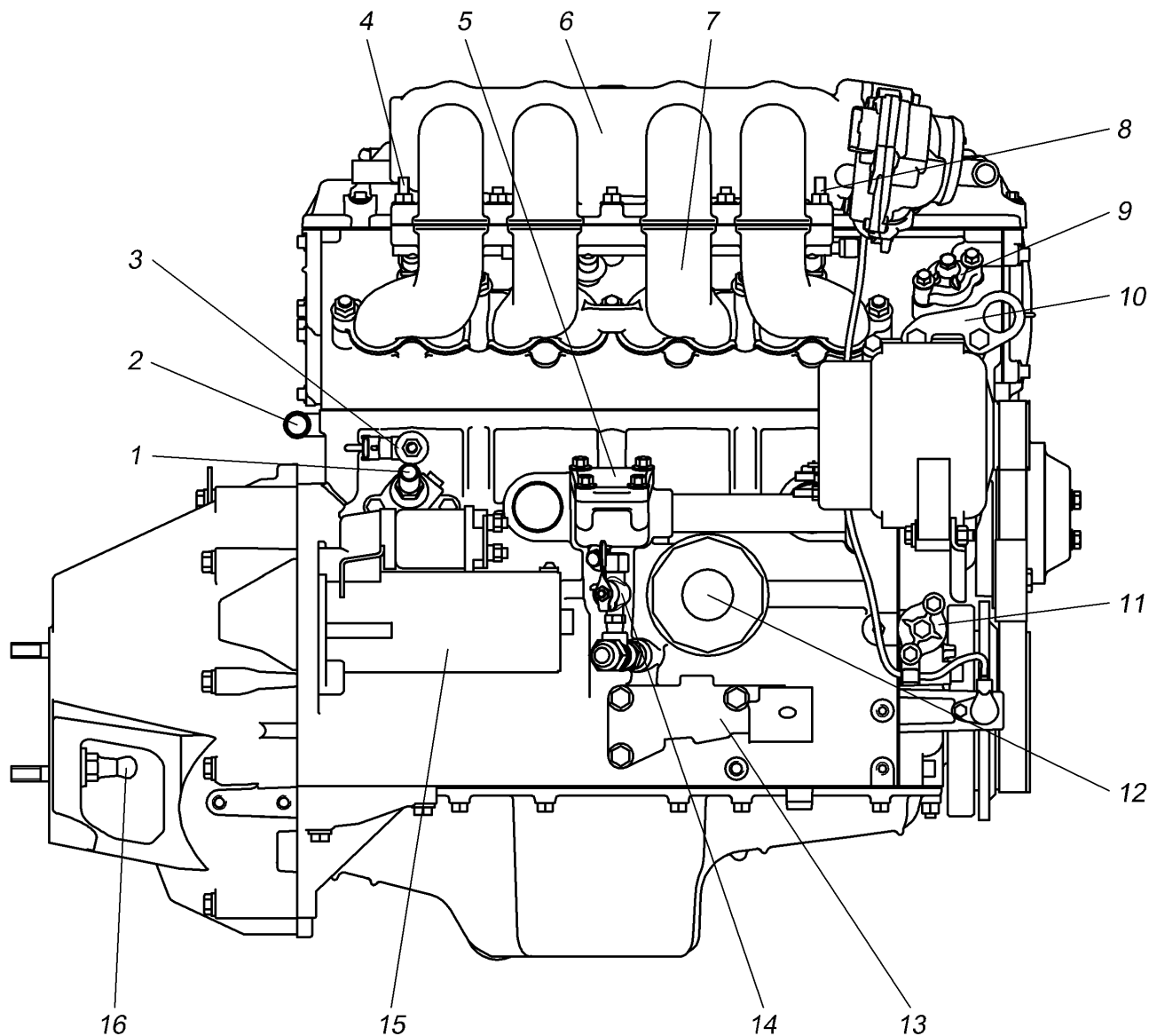
Рис.3. Вид двигателя справа:
