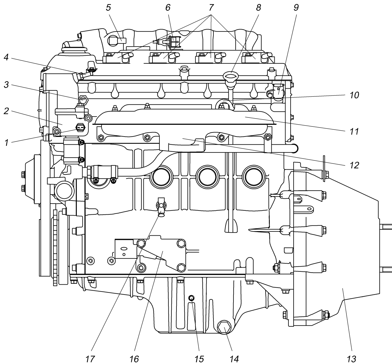
Рис.1. Левая сторона двигателя:
