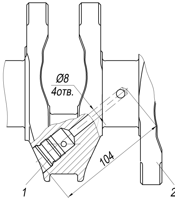
Рис.46. Удаление продуктов износа и нагара из полостей шатунных шеек коленчатого вала:
