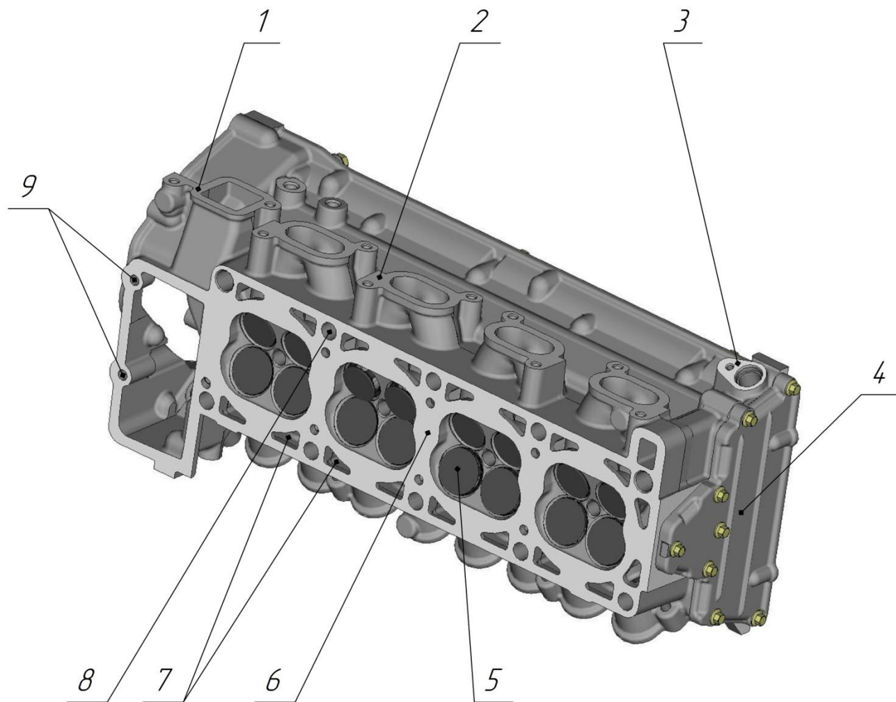
Рис.11. Головка цилиндров. Вид на камеры сгорания, на фланец выпускного коллектора и на заднюю крышку:
