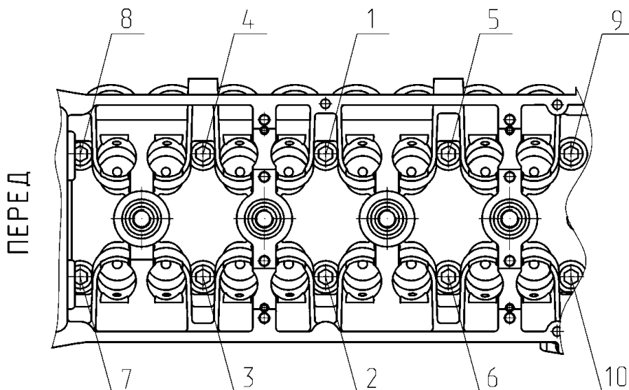
Рис.80. Последовательность затяжки болтов крепления головки цилиндров
