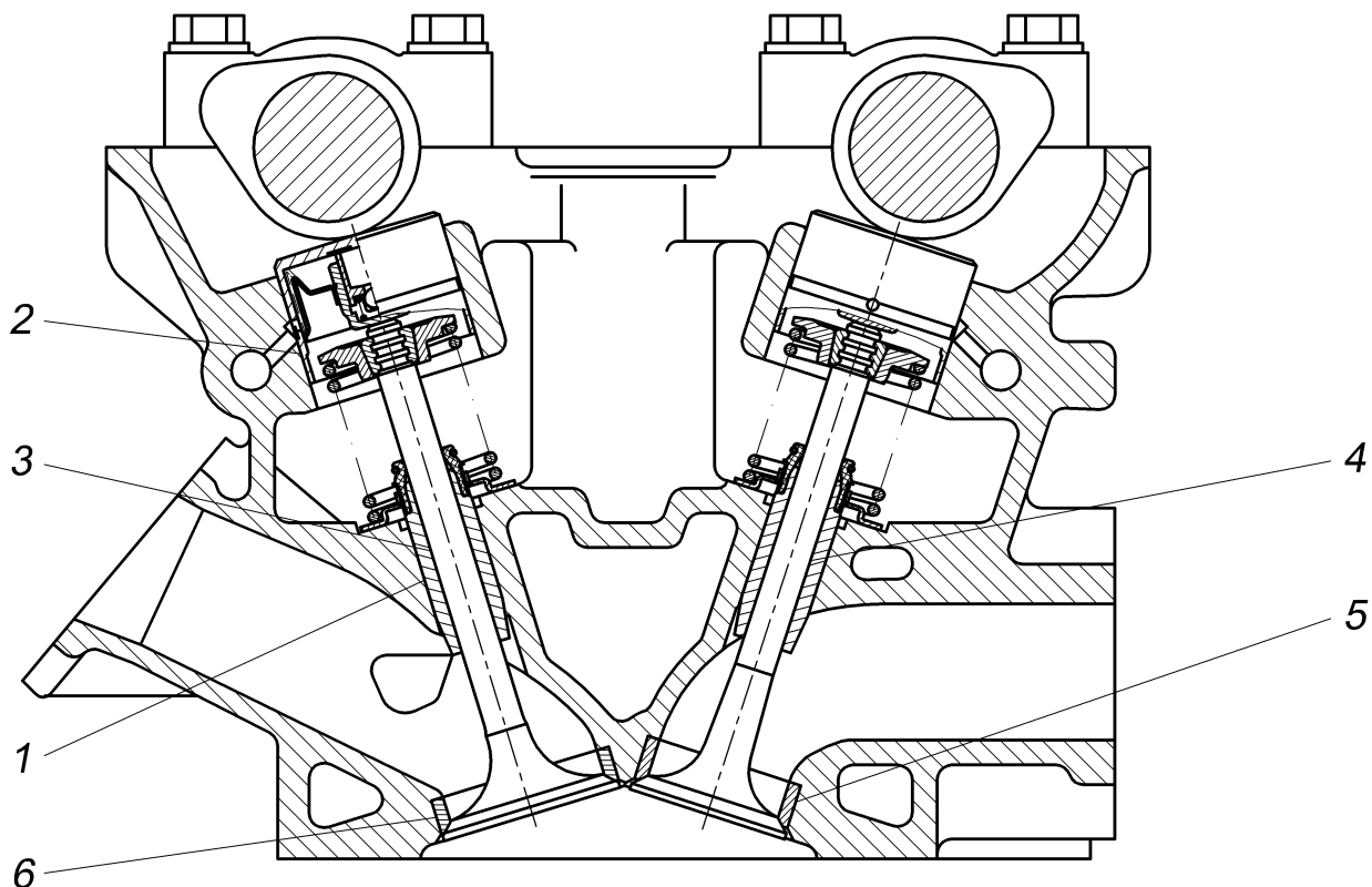
Рис.92. Привод клапанов
