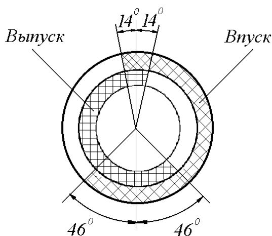
Рис.19. Фазы газораспределения
