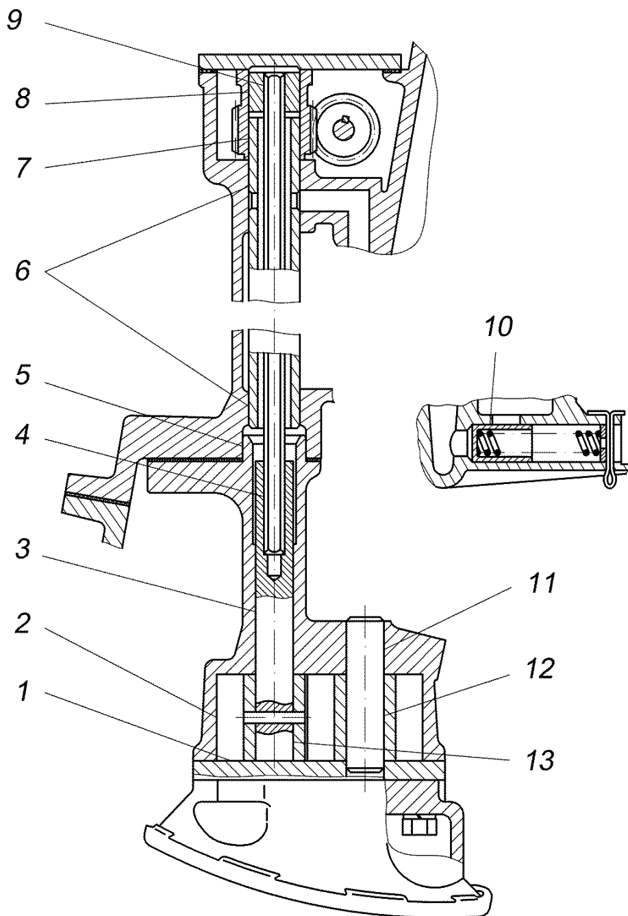
Рис.94. Масляный насос, редукционный клапан и привод масляного насоса
