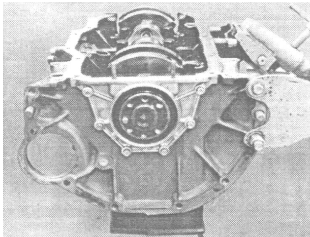
Рис.73. Установка сальниководержателя коленчатого вала
