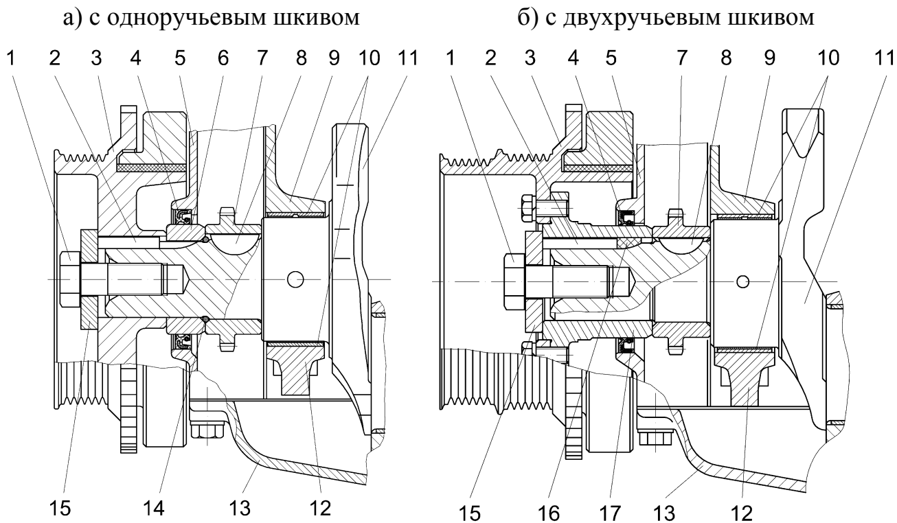
Рис.15. Передний конец коленчатого вала:
