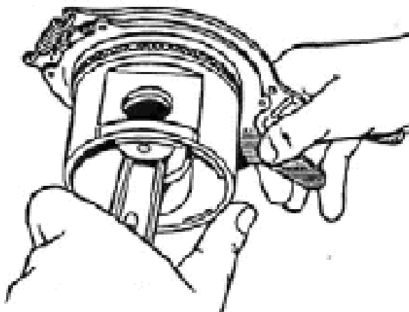
Рис.78. Установка поршневых колец на поршень
