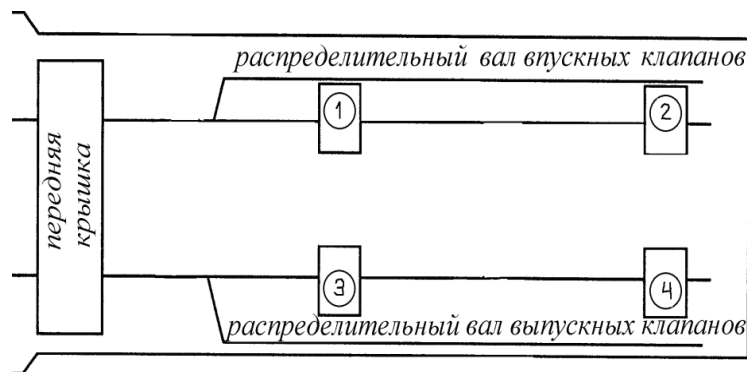
Рис.82. Схема установки крышек распределительных валов
