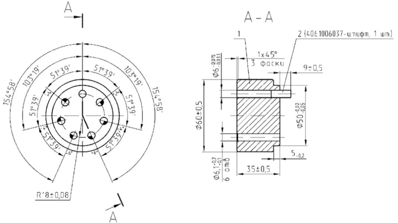
Рис.55. Кондуктор для сверления дополнительных отверстий под штифт в звездочках распределительных валов
