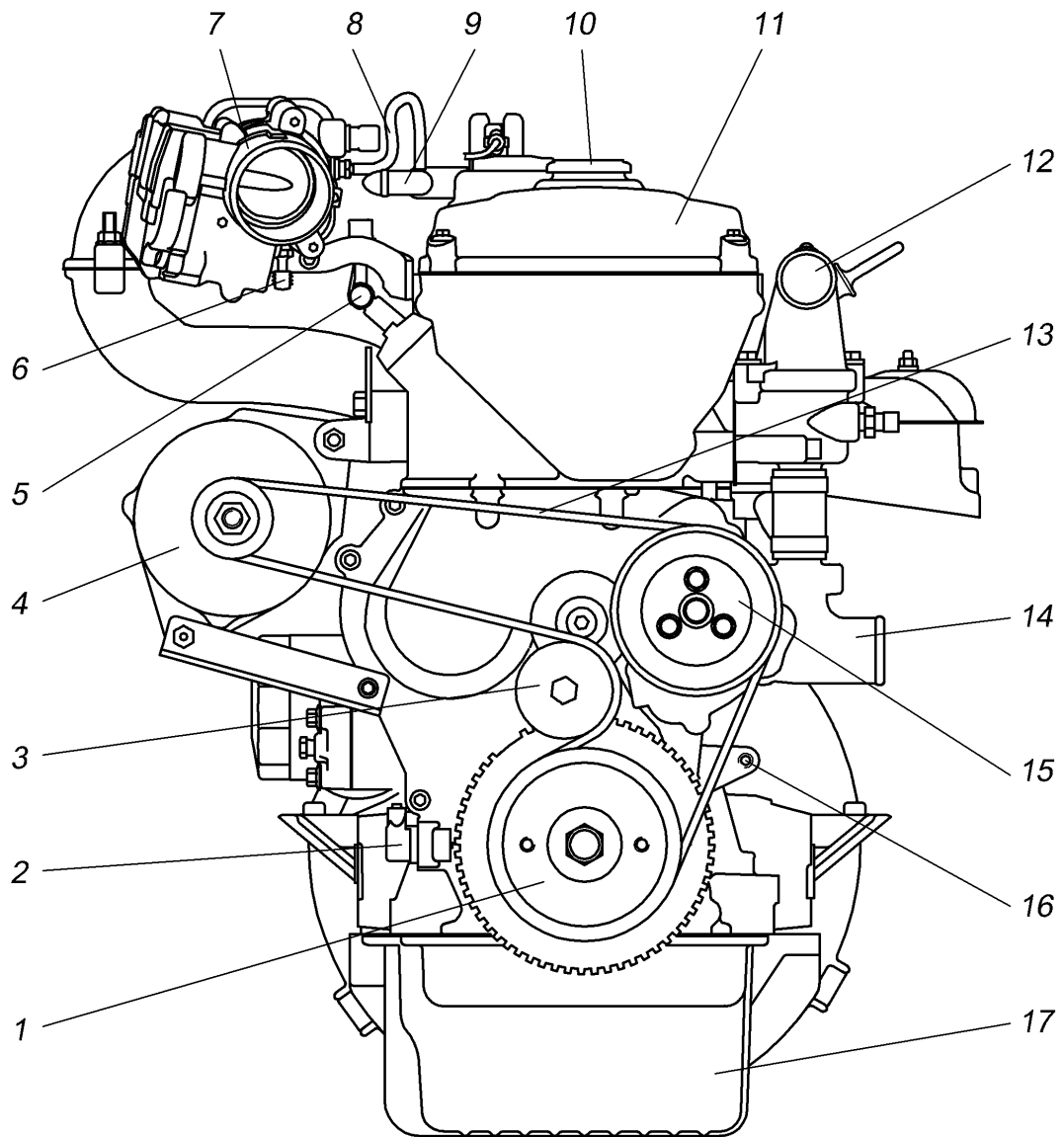
Рис.2. Вид двигателя спереди:
