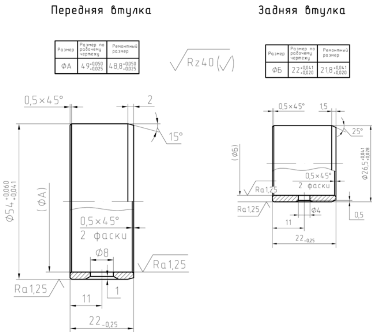
Рис.45. Ремонтные втулки опор промежуточного вала
