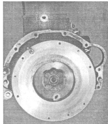
Рис.74. Установка маховика
