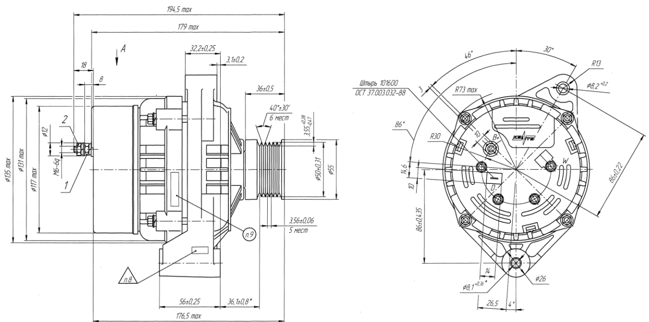
Рис.41. Габаритные размеры и токоскоростная характеристика генератора 9422.3701-10 ОАО «ЗиТ»
