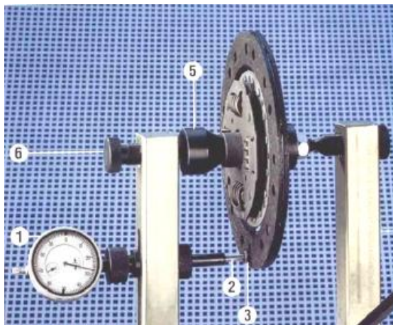
Рис.87. Проверка биения рабочей поверхности ведомого диска
