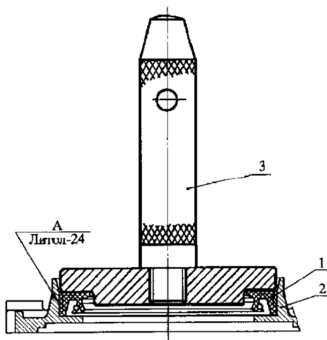
Рис.72. Запрессовка сальника в сальникодержатель:
