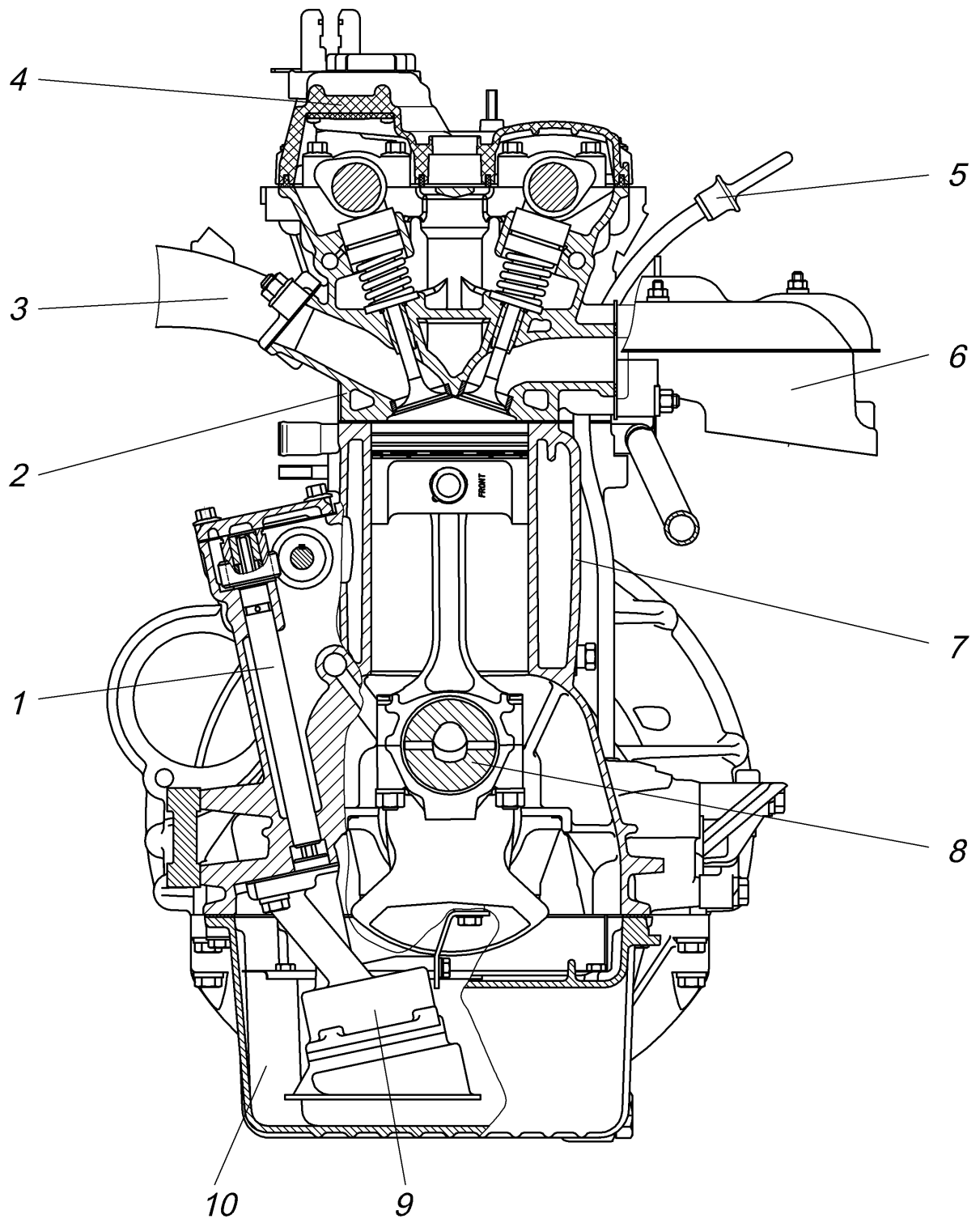
Рис.4. Поперечный разрез двигателя:
