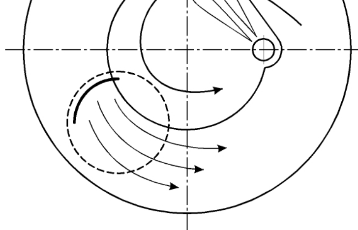
Рис. 6. 33. Полуразделённая камера сгорания с плёночным смесеобразованием
